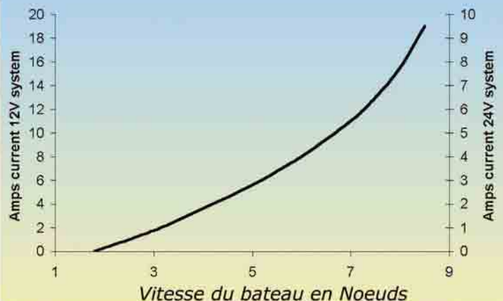
Performances mode hydrogénérateur
